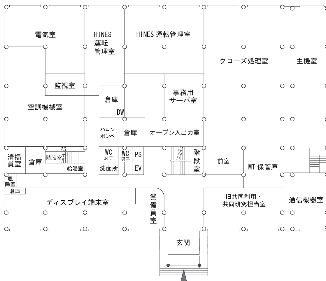
北館 1 階平面図
