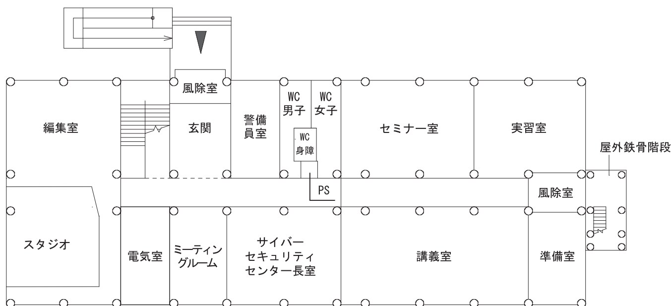
南館 1 階平面図
